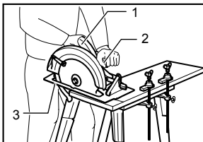
1. Poignée arrière 2. Poignée avant 3. Base
