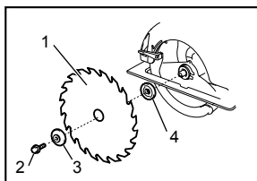
1. Lame 2. Boulon hexagonal 3. Bague externe 4. Bague interne
