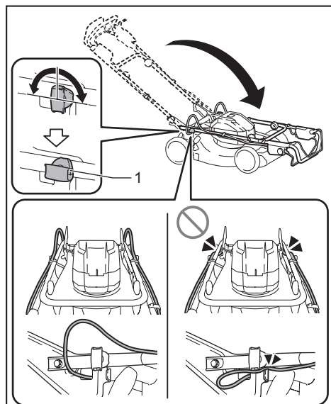
► 1. Knob
