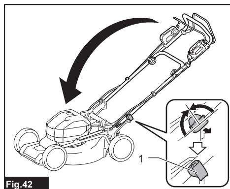
► 1. Knob
